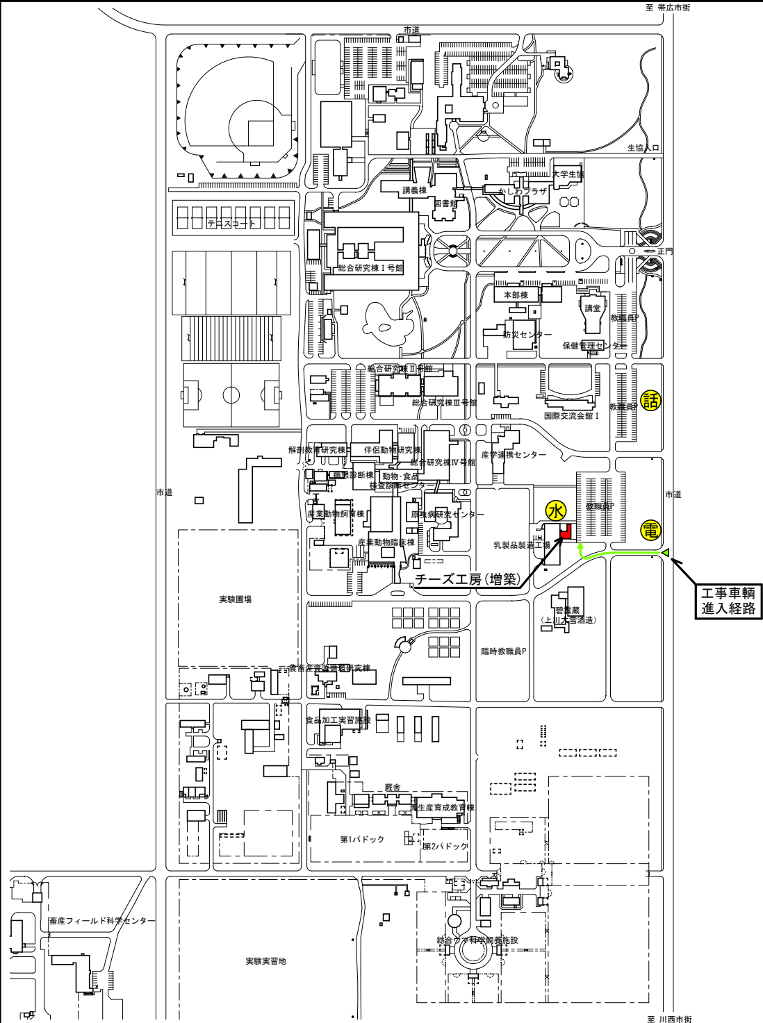
構内配置図 S=1/6,000 (A-4)
