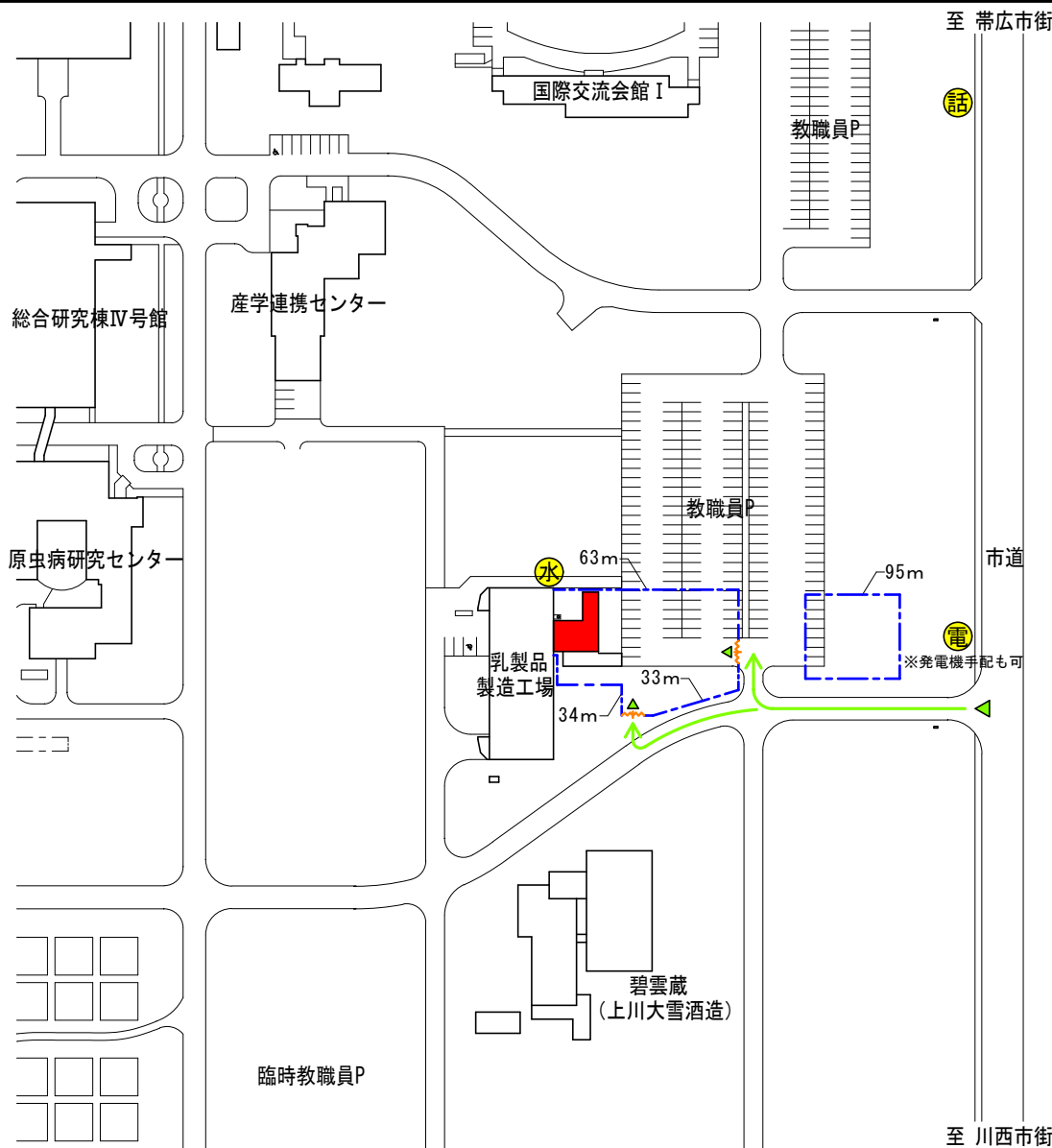
工事配置図 S=1/2,000 (A-4)
