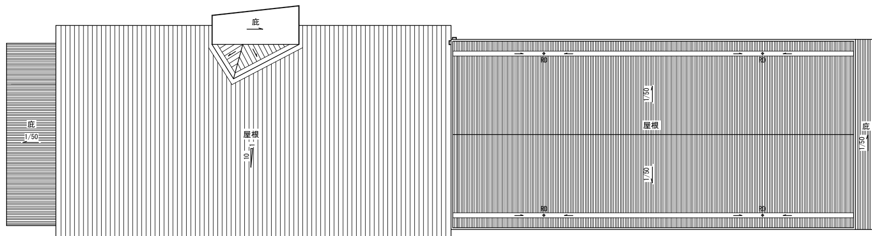
実習管理棟・屋根伏図
