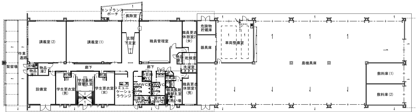
実習管理棟・1階平面図
