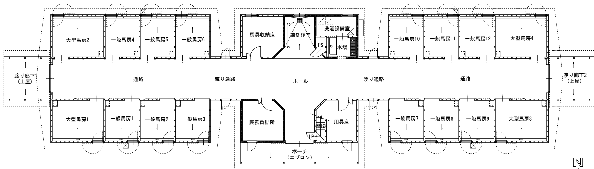
1階平面図
