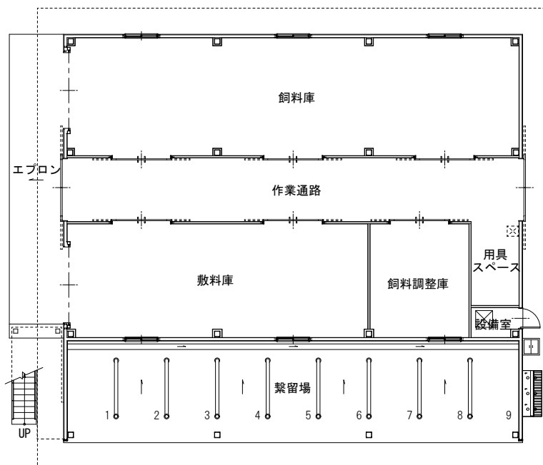
1 階平面図
