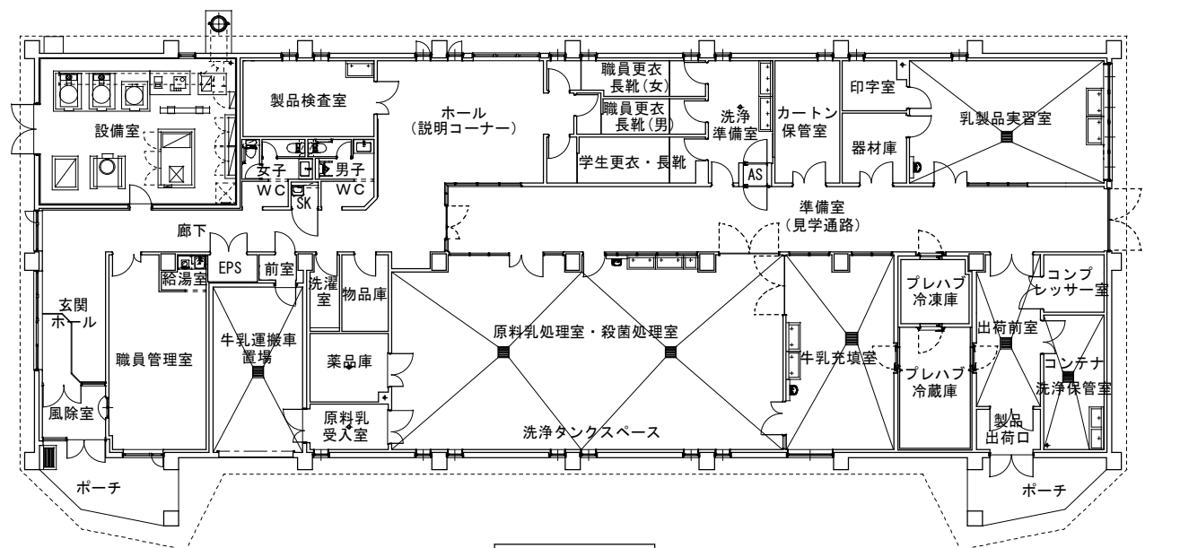
1 階平面図
