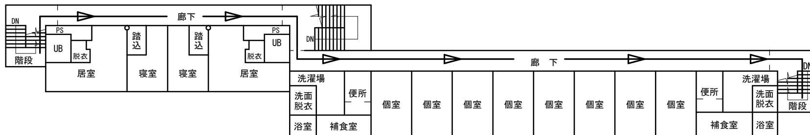
4 階平面図
