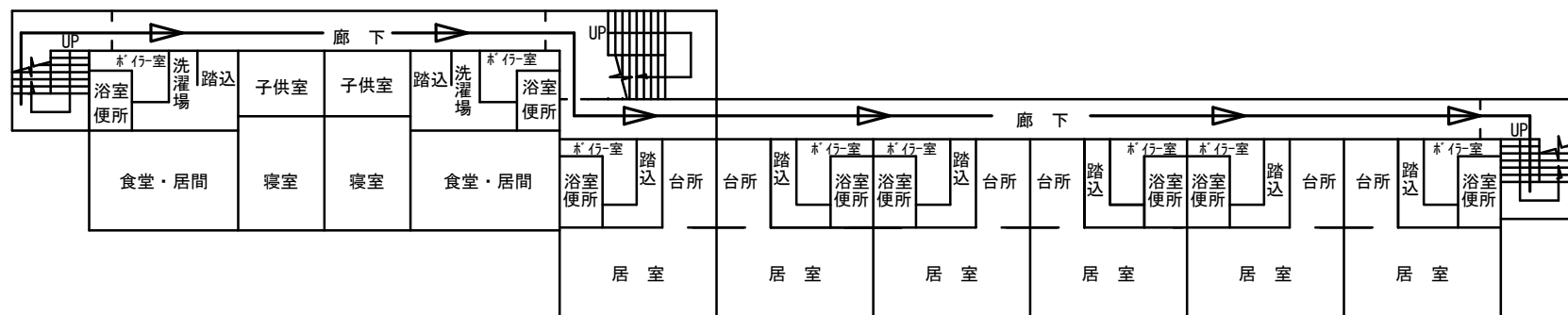
2 階平面図
