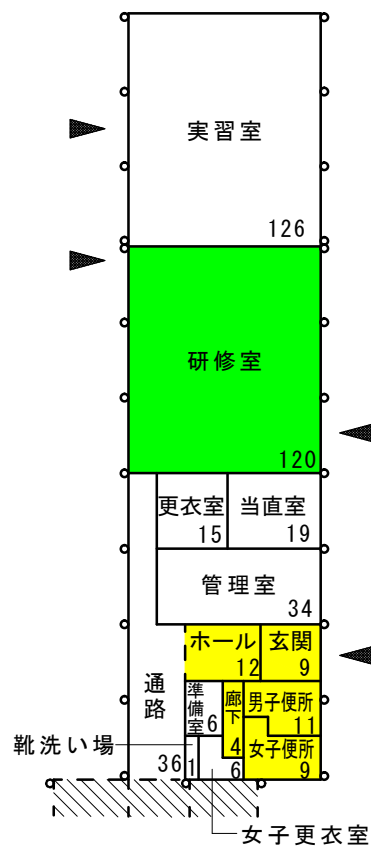
畜産フィールド科学センター 牛群管理棟 1階平面図 S = 1 / 4 0 0
