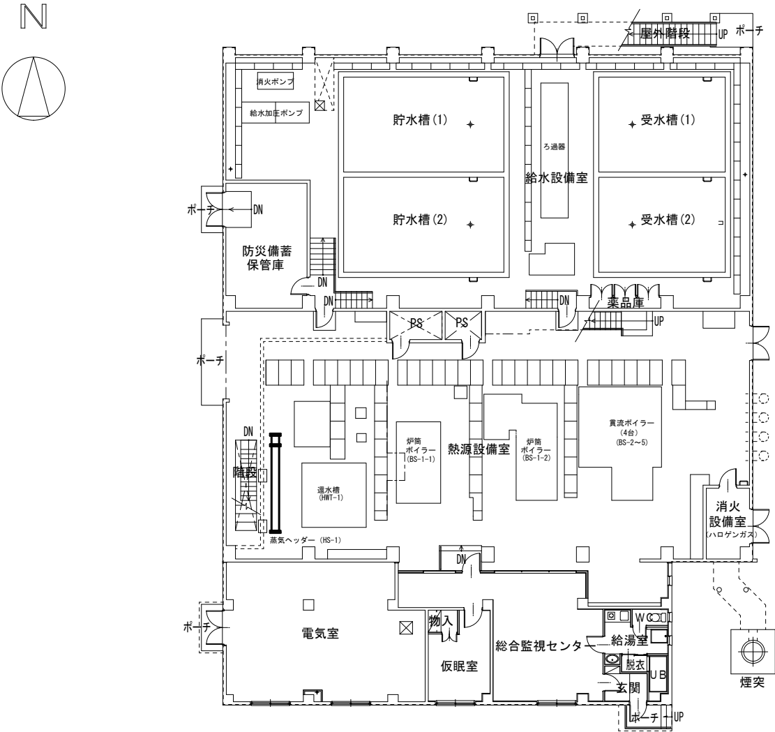
防災センター平面図
