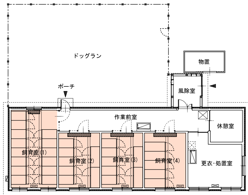
改修前・平面図
