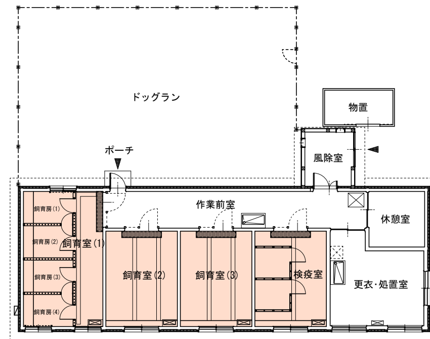
改修後・平面図
