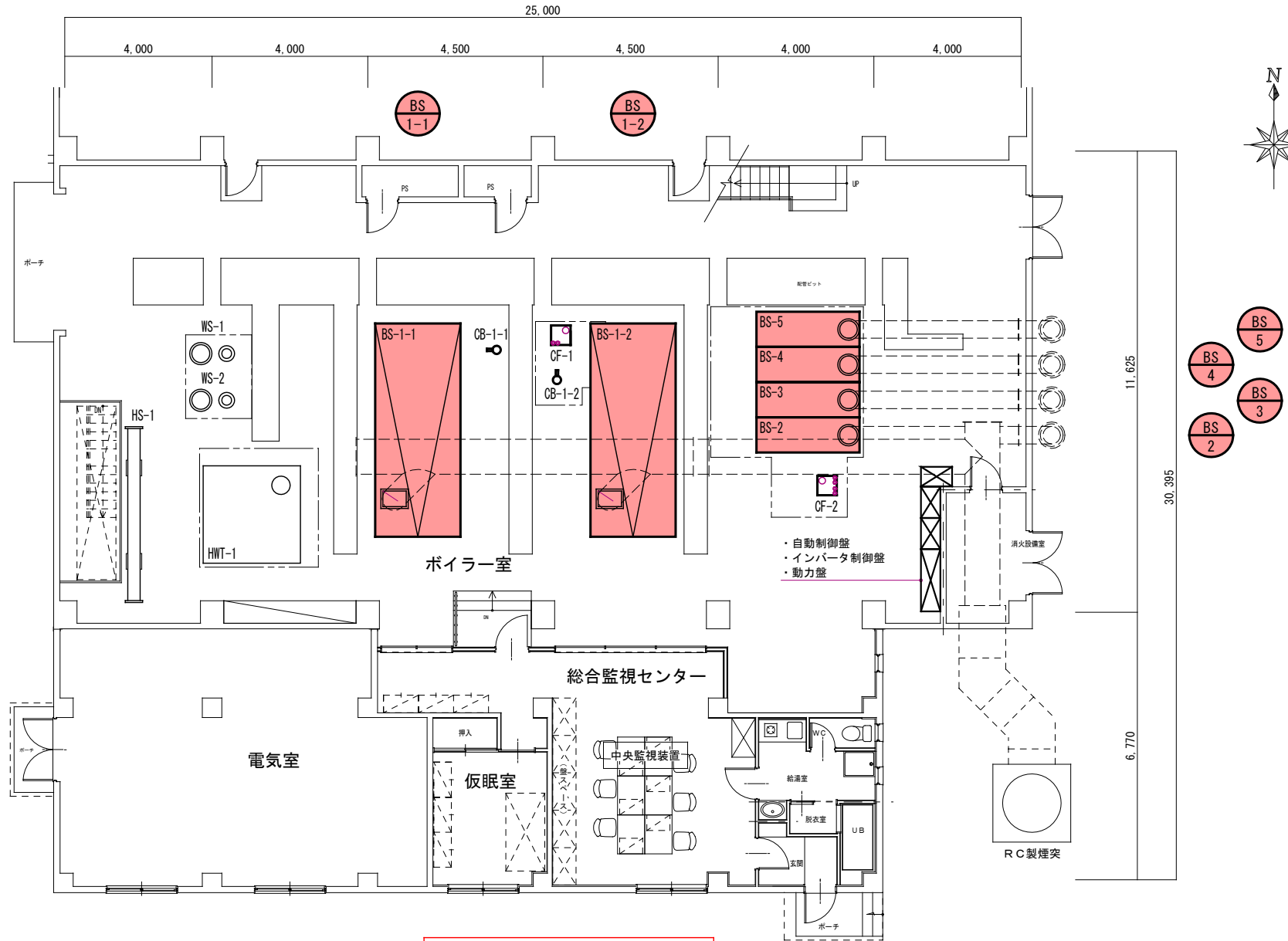
中央機械室平面図 S=1:150
