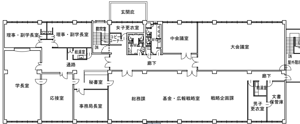
増築/改修前・2階平面図
