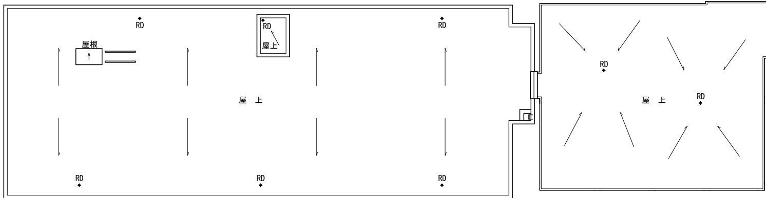
増築/改修後・屋上伏図
