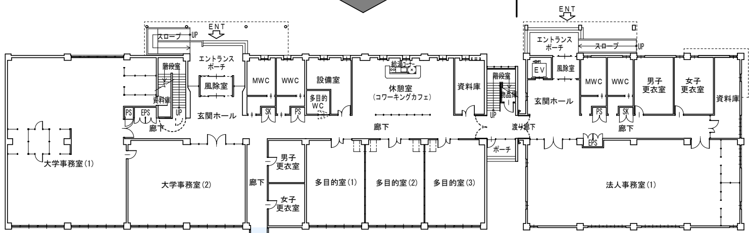
増築/改修後・1階平面図
