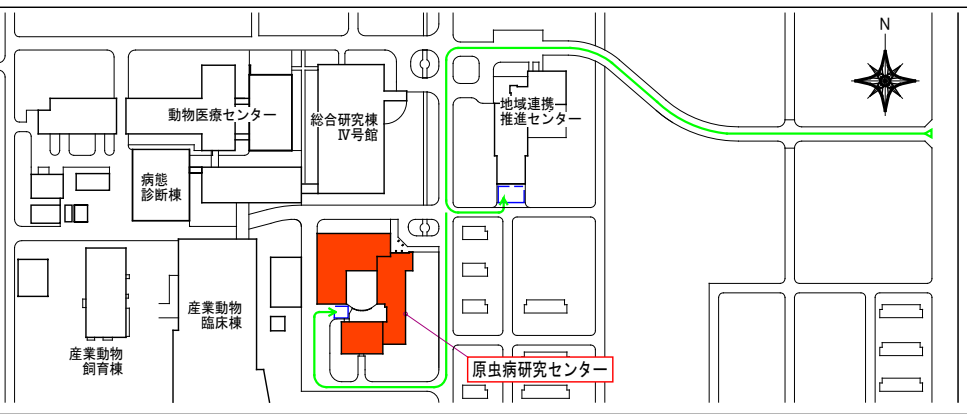
工事配置図
