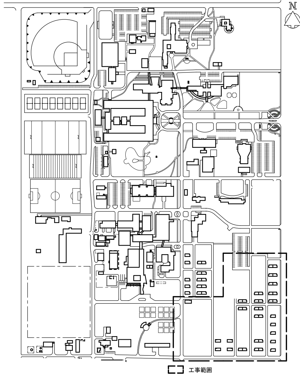
工事位置図
