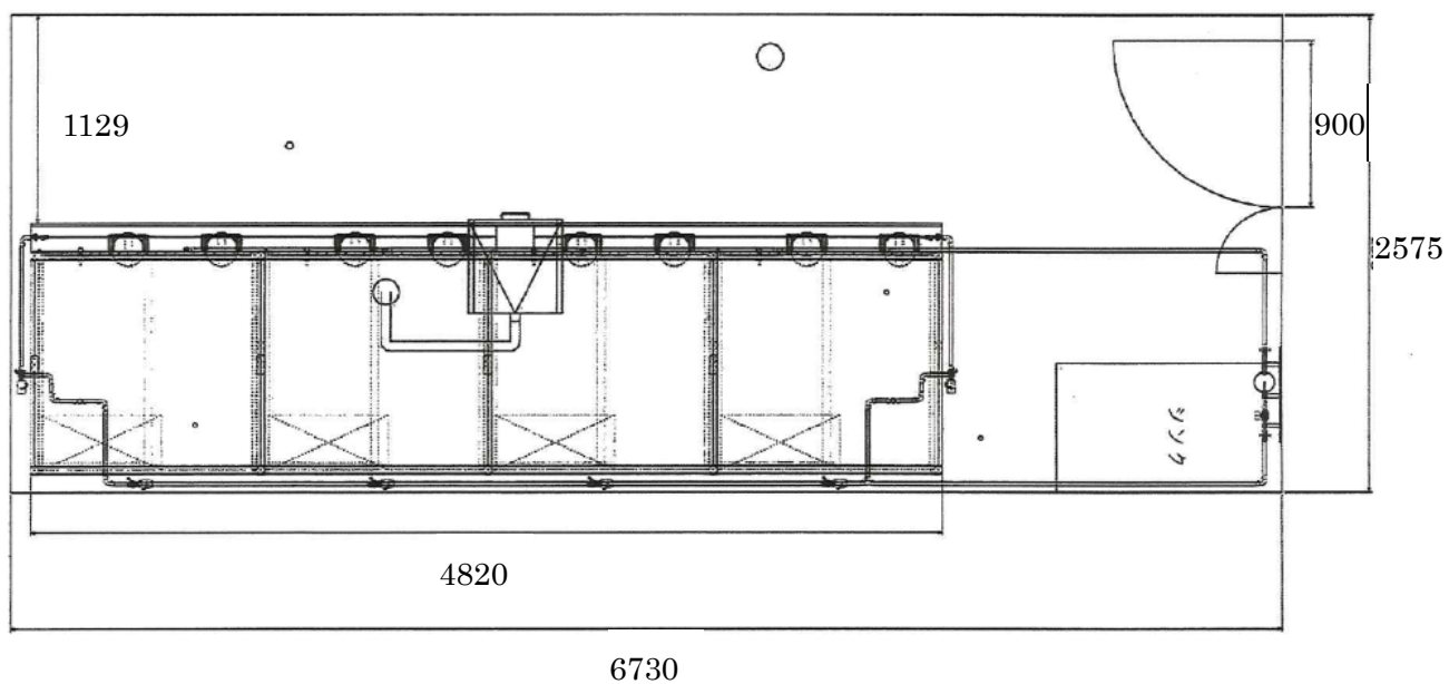
図面名称：原虫病研究センター3階318室
