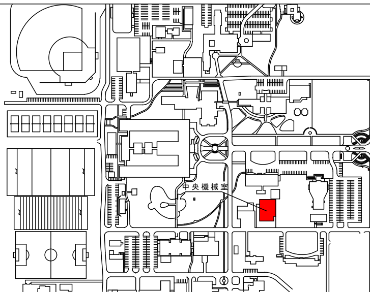
工事配置図
