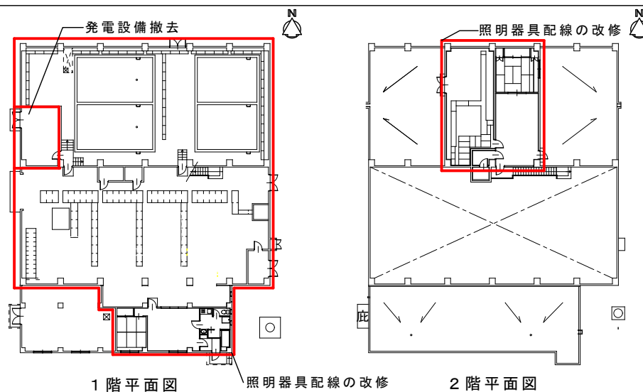
中央機械室 改修後
