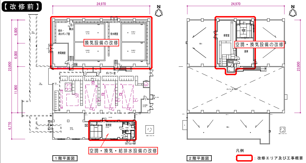
工事概要 / 平面図
