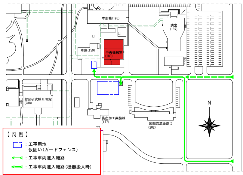
工事配置図
