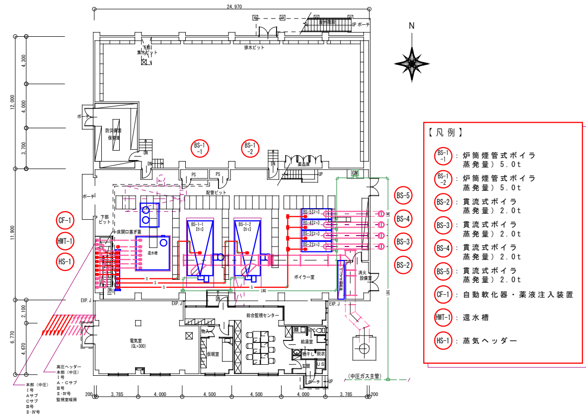
平面図
