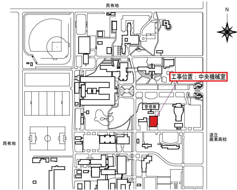
工事配置図
