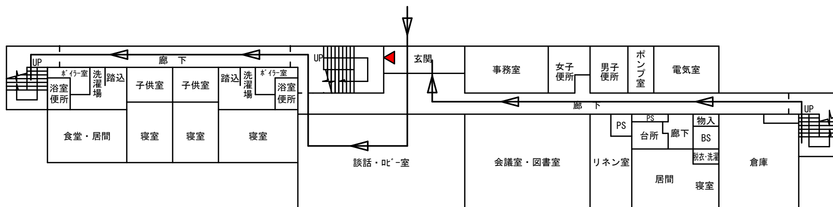
2 階平面図
