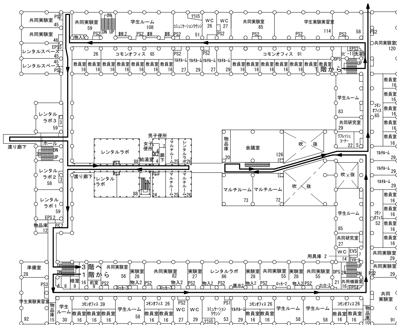
総合研究棟 I 号館 2 階平面図
