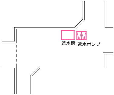
Cサブステーション平面図
