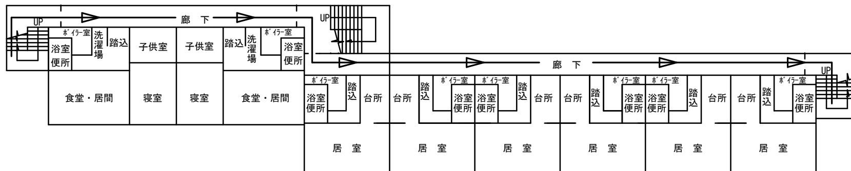
2 階平面図
