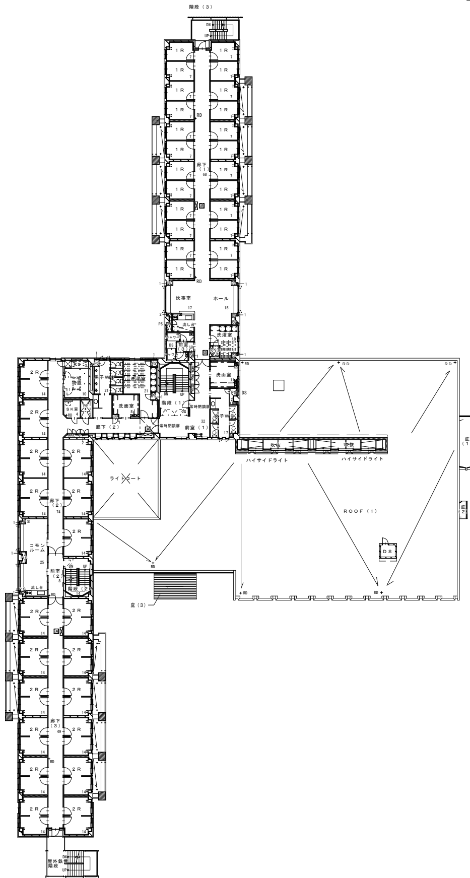
学生寄宿舍 2階平面図
