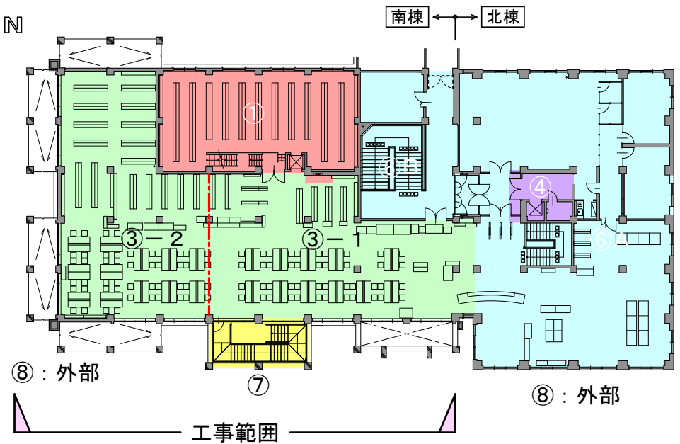
改修前・2階平面図
