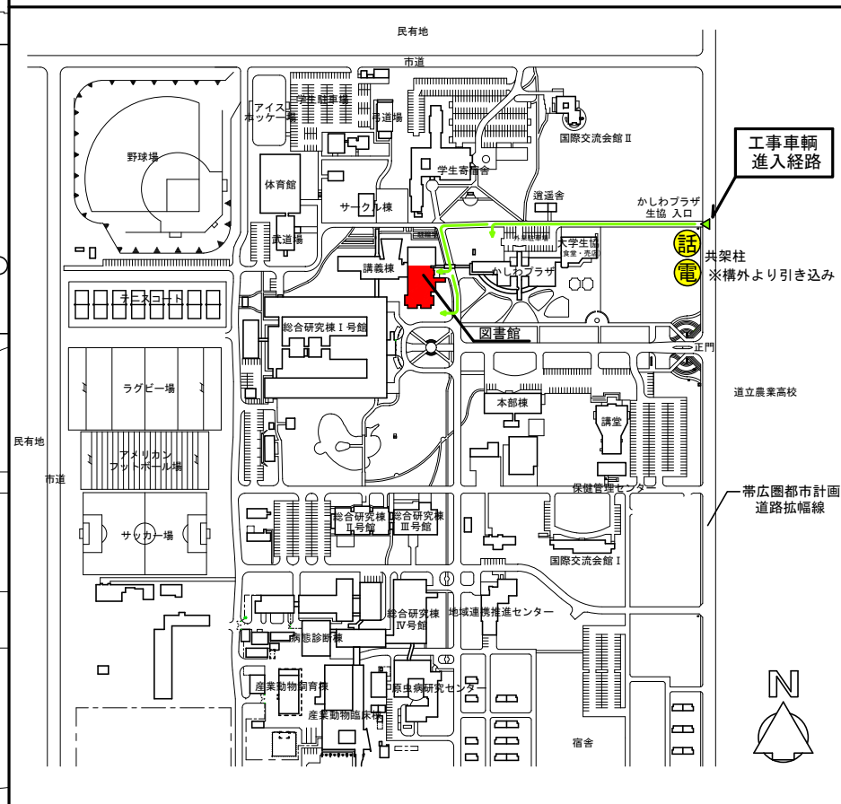
配置図 S=1/6,000 (A-4)
