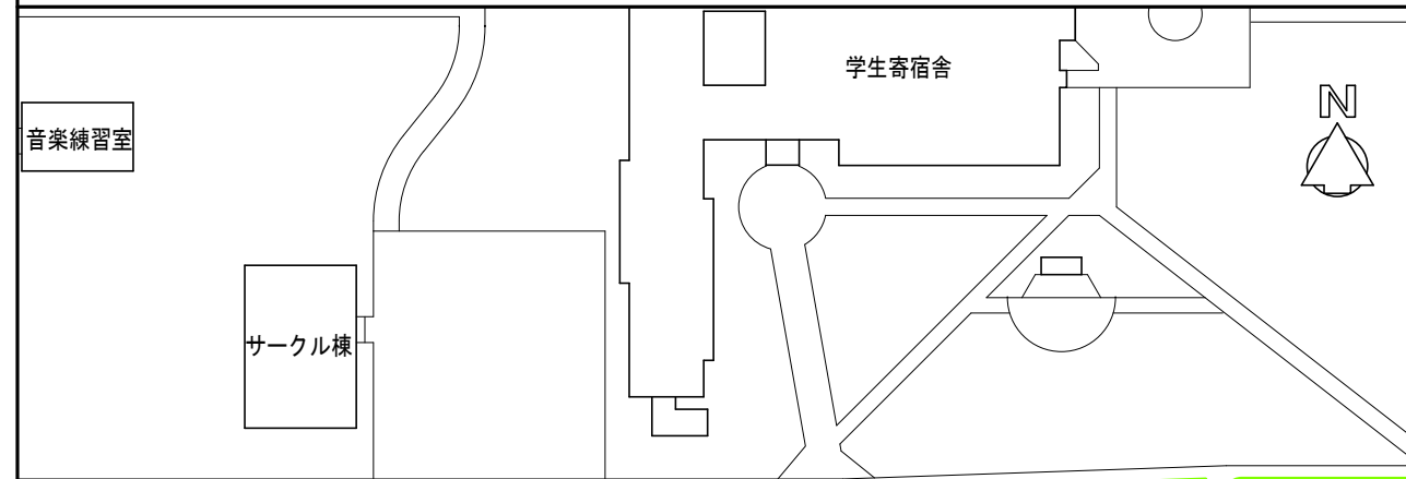
工事配置図 S=1/1,000 (A-4)
