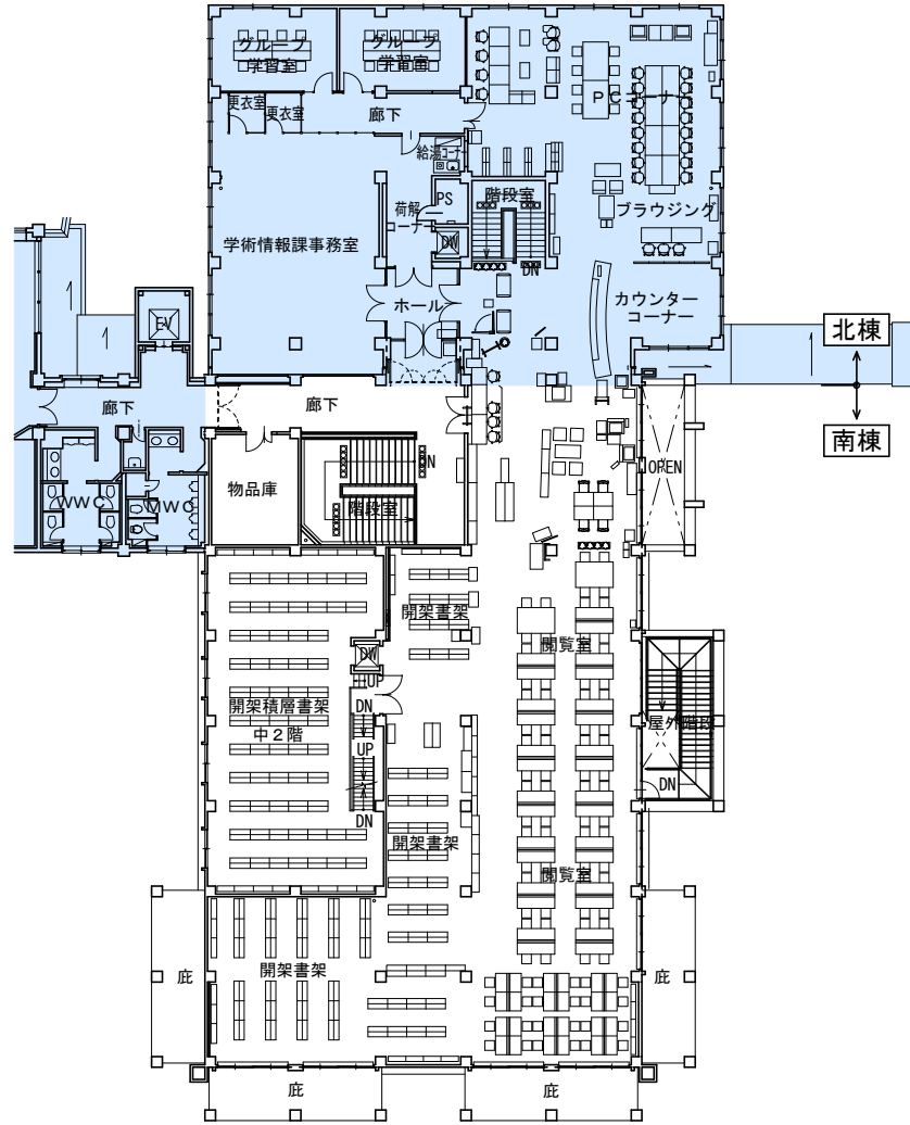
改修前・2階平面図
