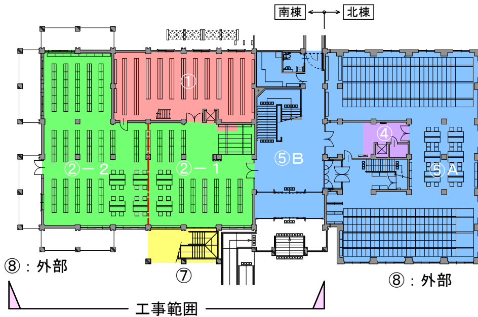
改修前・1階平面図
