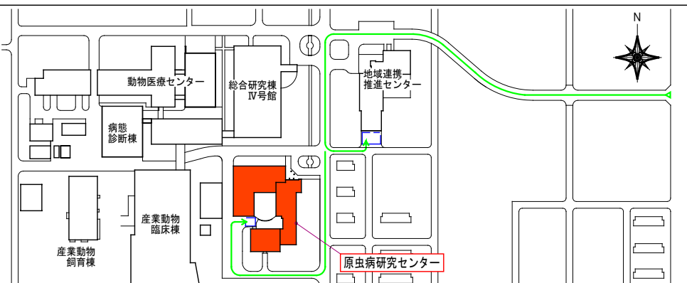
工事配置図
