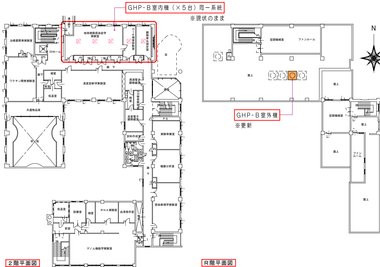
工事配置図
