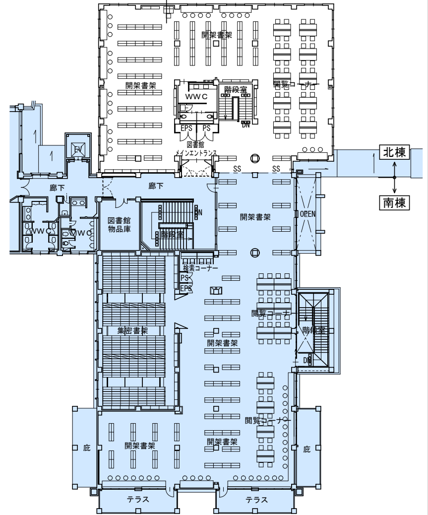
改修後・2階平面図
