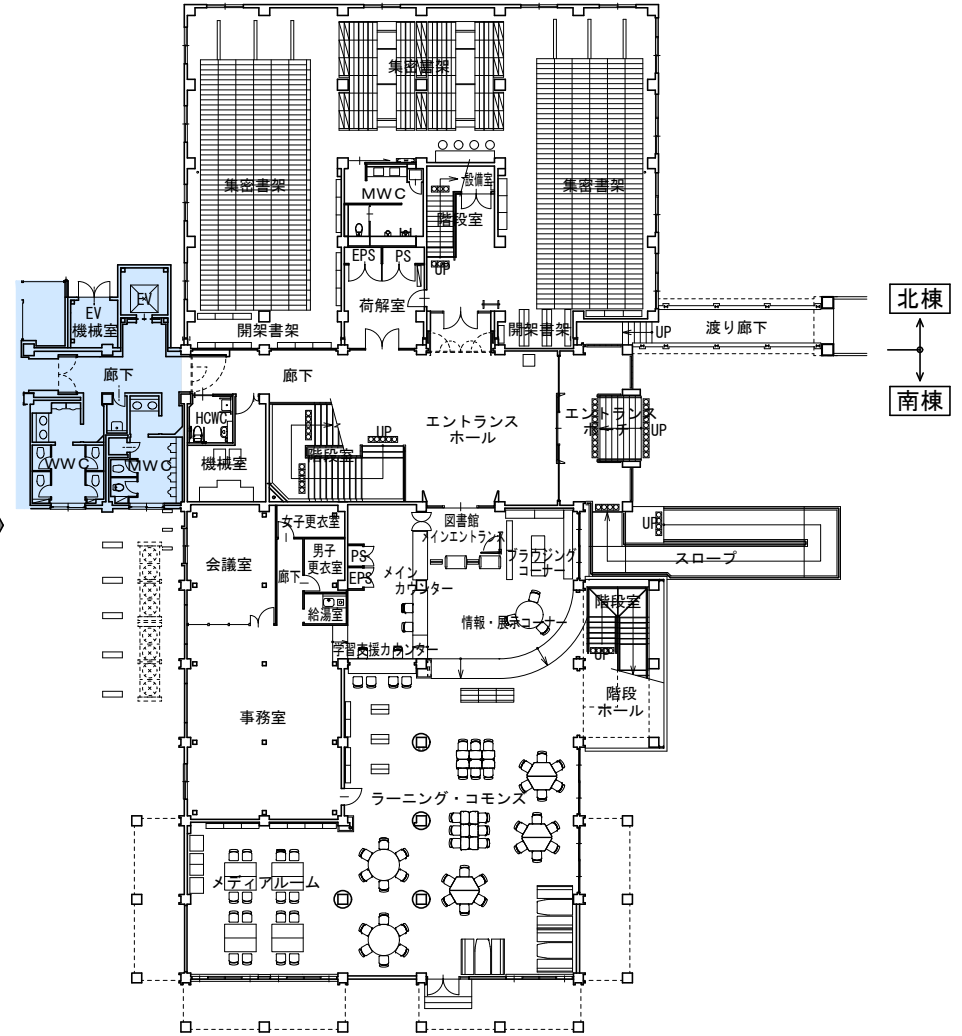
改修後・1階平面図
