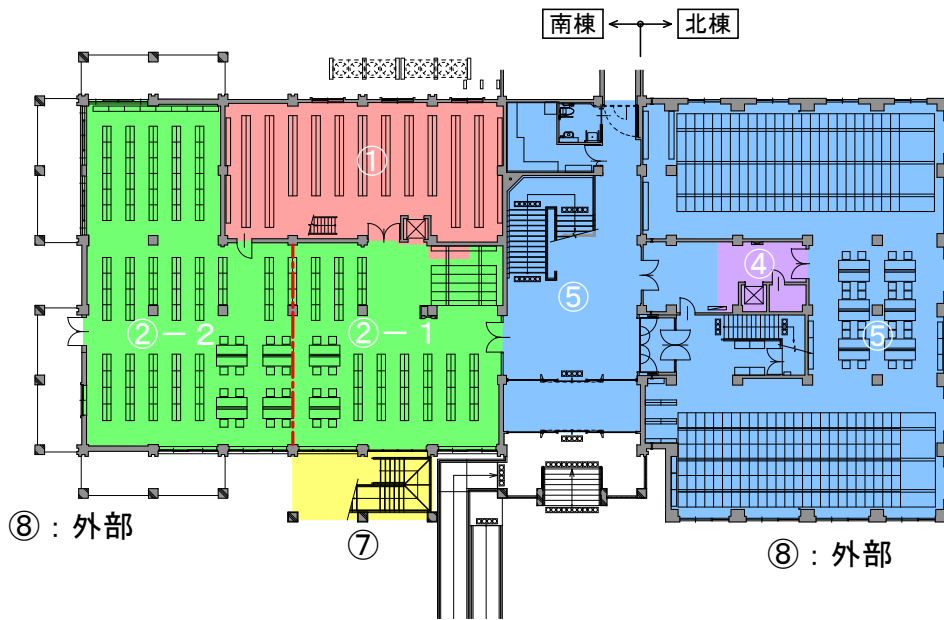
改修前・1階平面図
