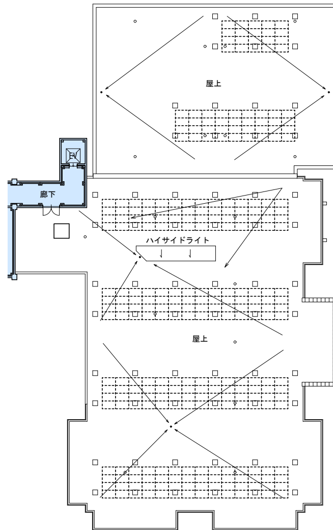
改修後・屋上平面図
