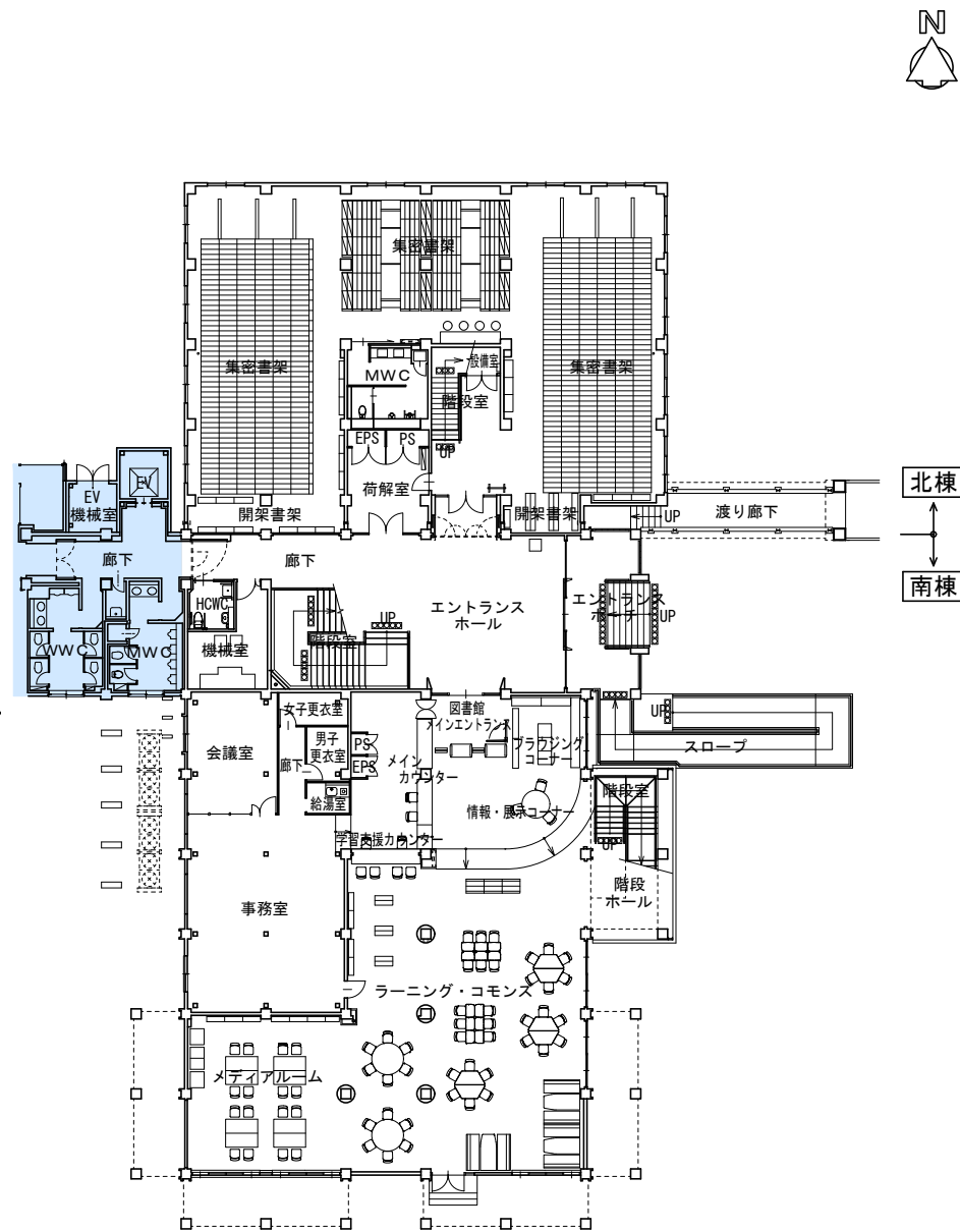
改修後・1階平面図
