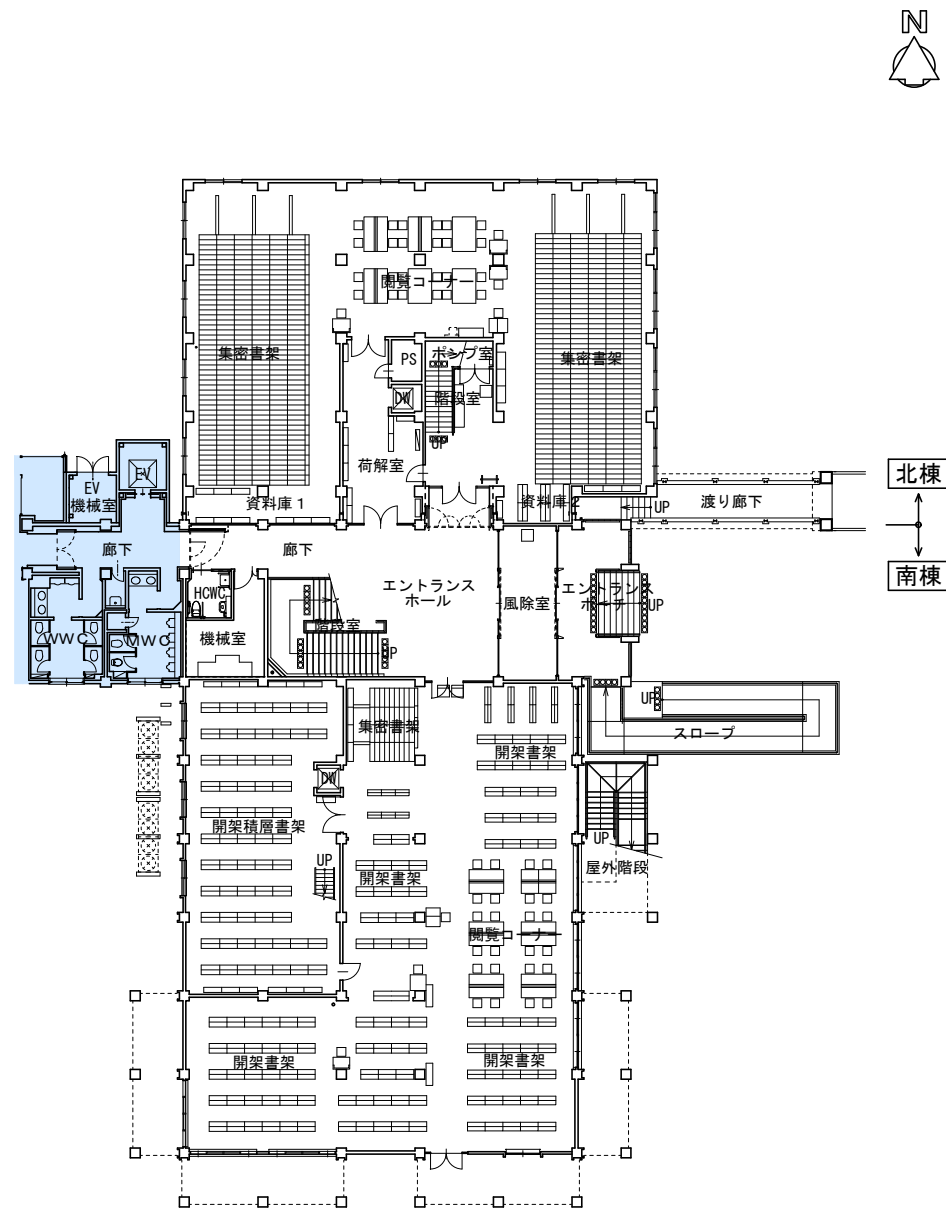
改修前・1階平面図
