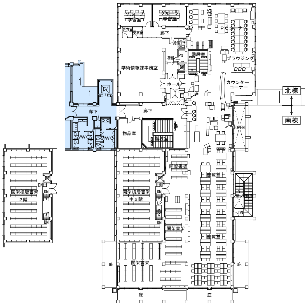
改修前・2階平面図
