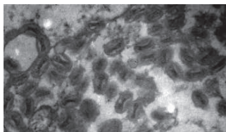
ボックスウイルスの電子顕微鏡写真
