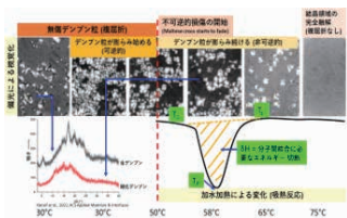
デンプンの膠化機構
