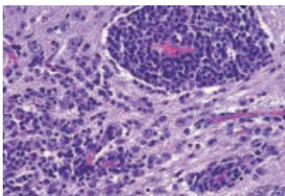
ネオスポラによる牛の脳炎 (HE染色)
