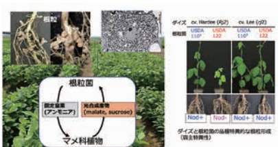
根粒菌のマメ科植物との共生相互作用とその宿主特異性
