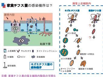
ネズミチフス菌と家禽チフス菌の感染機序の比較
