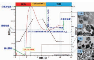
デンプンのゲル化とゲル特性
